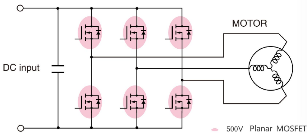
高速电吹风筒拓扑
