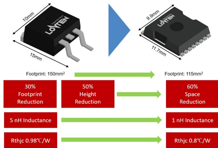
图2 TOLL 与 TO-263-2L 封装对比图
