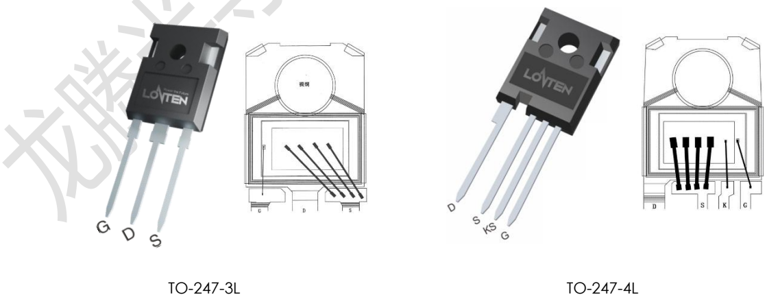
图3 TO-247-3L 与 TO-247-4L 封装对比图
