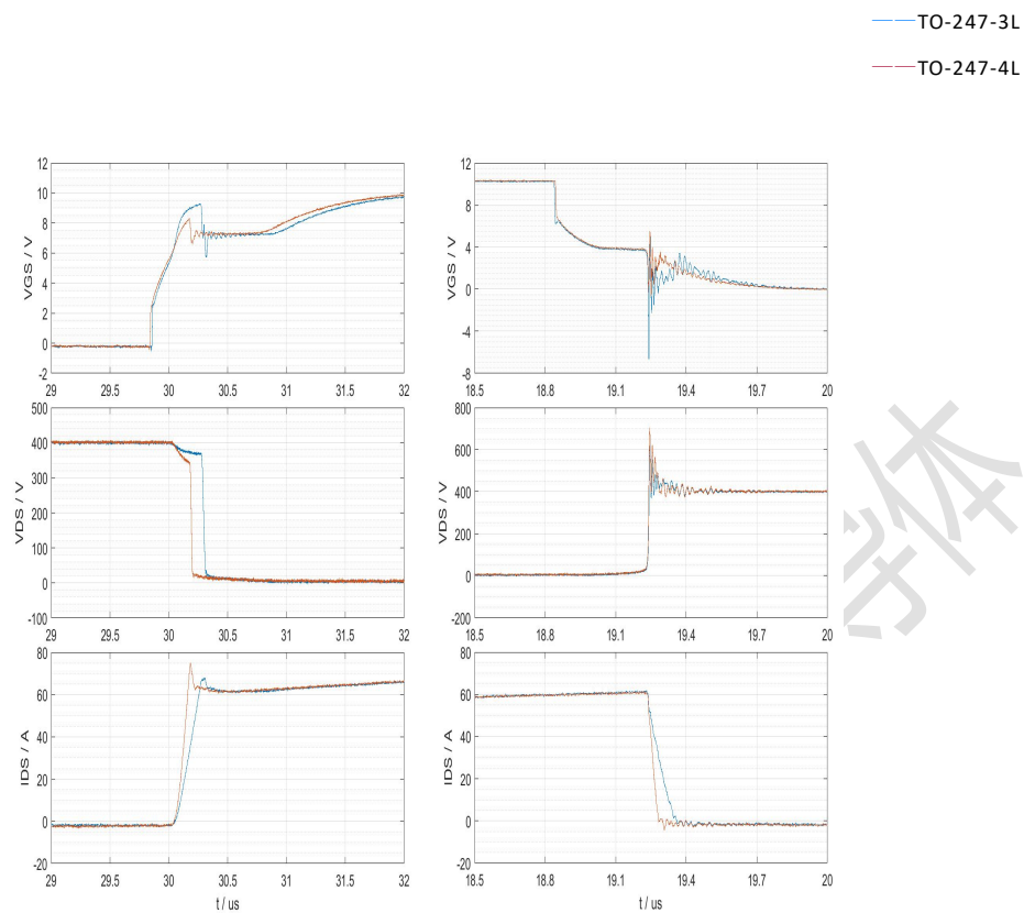
图 6 TO-247-3L 与 TO-247-4L 开关波形对比图
