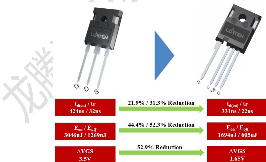
图 5 TO-247-3L 与 TO-247-4L 封装对比图
